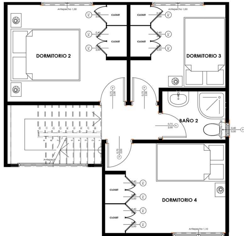
Planta Segundo Piso 38,56 m 2
