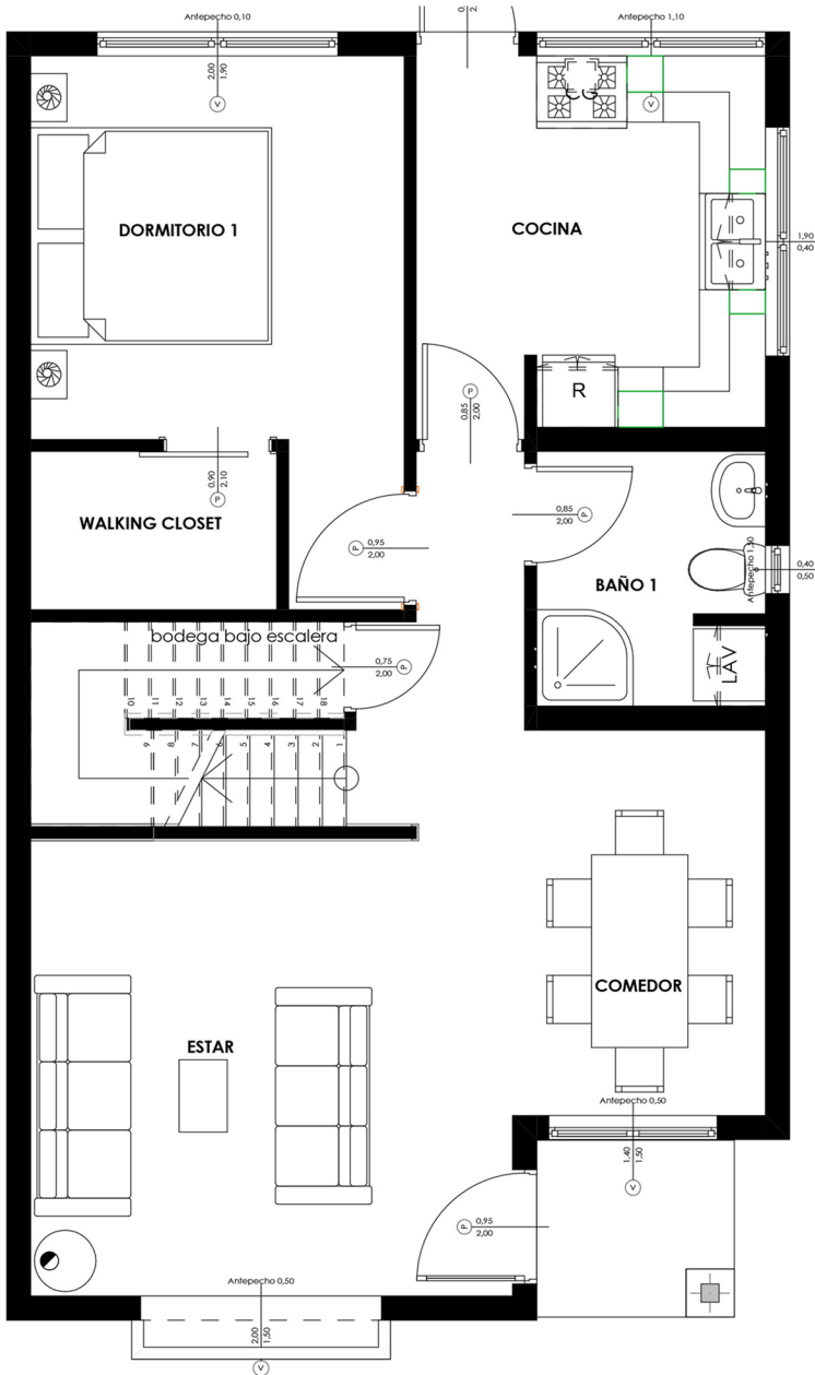
Planta Primer Piso 68,86 m 2
